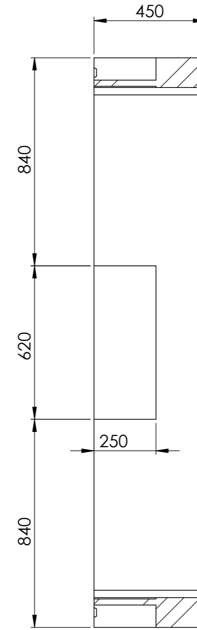
SCHNITT A-A MABSTAB 1 : 15
